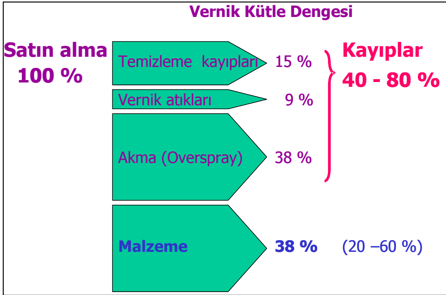
Resim 3.2: Tipik bir vernikleme işlemi için kütle dengesi örneği Kaynak; Wilfried Denz, www.denz-unweltberatung.de
